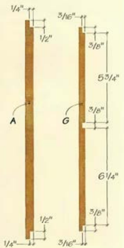
GROOVE LAYOUTS
