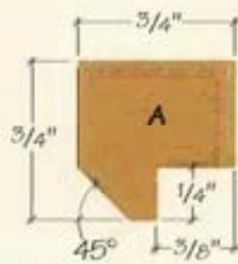
DETAIL: FRAME
